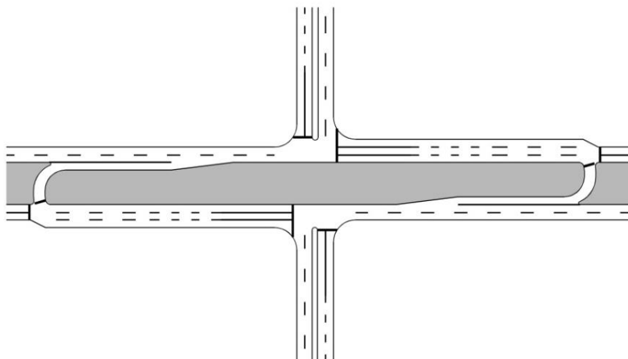
Рисунок 17 – Схема пересечения с отнесенными левыми поворотами с центральной разделительной полосой без прямого проезда второстепенного направления
