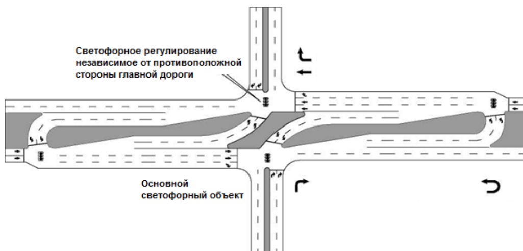
Рисунок 21 – Пересечение в одном уровне с отнесенными левыми поворотами с второстепенной дороги и левым поворотом с главной дороги без обеспечения прямого проезда по второстепенному направлению
