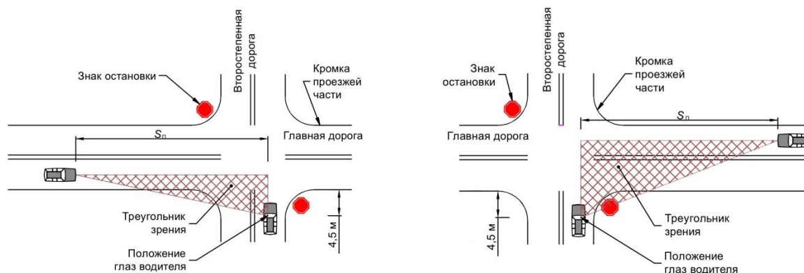
Рисунок 2 – Схема к определению минимального расстояния видимости для остановки S_{п} на нерегулируемом пересечении с обязательной остановкой
