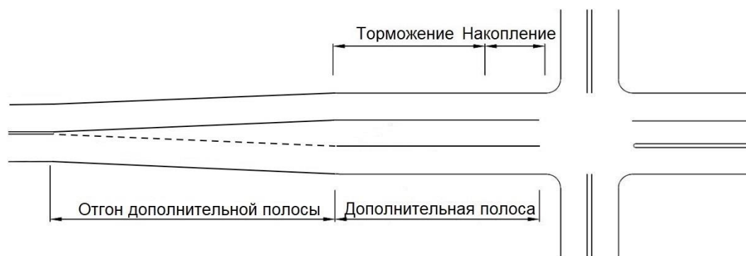
Рисунок 12 – Принципиальная схема отгона полосы для поворота налево на главной дороге
