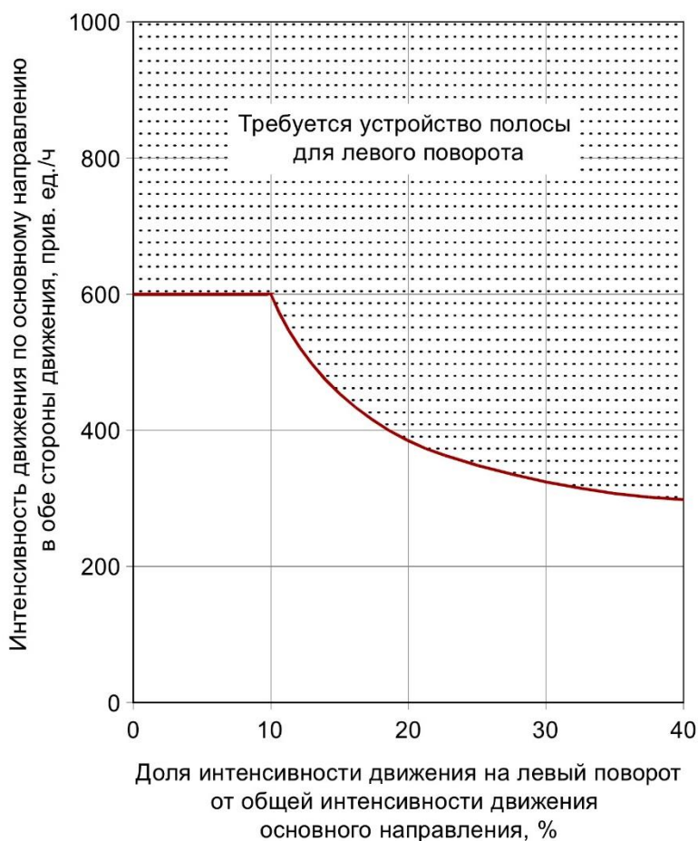
Рисунок 8 – Диаграмма для определения необходимости полосы для левого поворота
