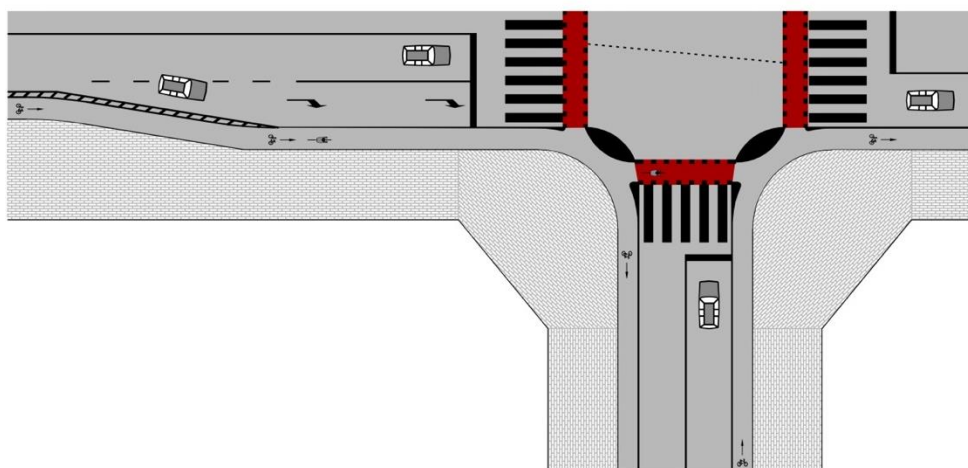
Рисунок 26 – Пример расположения велосипедной полосы относительно полосы для поворота направо
