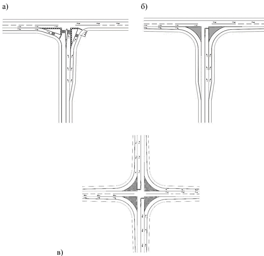
Рисунок 3 – Организация движения на нерегулируемом примыкании (а,б) и пересечении (в) в одном уровне с двухполосной второстепенной дорогой с полосой для поворота налево на главную дорогу
