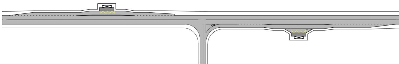
Рисунок 28 – Пример расположения автобусных остановок вблизи примыкания
