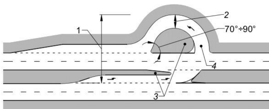
Рисунок 19 – Схема пересечения в одном уровне с отнесенными левыми поворотами с недостаточной для разворота шириной центральной разделительной полосы
