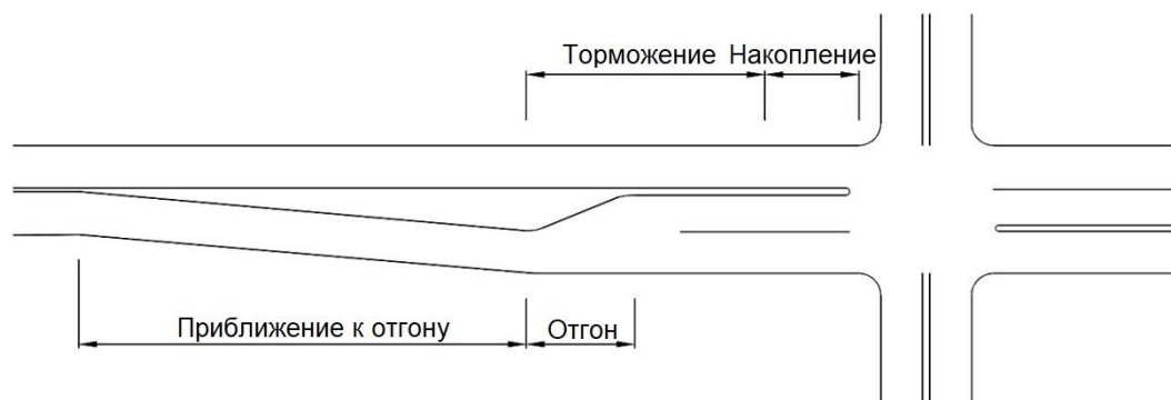
Рисунок 10 – Принципиальная схема отгона полосы для поворота налево на главной дороге
