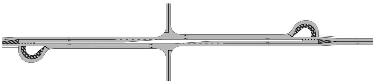
Рисунок 18 – Схема нерегулируемого пересечения с отнесёнными разворотами без центральной разделительной полосы
