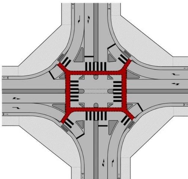
Рисунок 23 – Совмещение пешеходных путей и велосипедных дорожек
