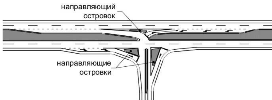
Рисунок 14 – Пример устройства полосы для поворота налево на примыкании при наличии центральной разделительной полосы с устройством направляющих островков
