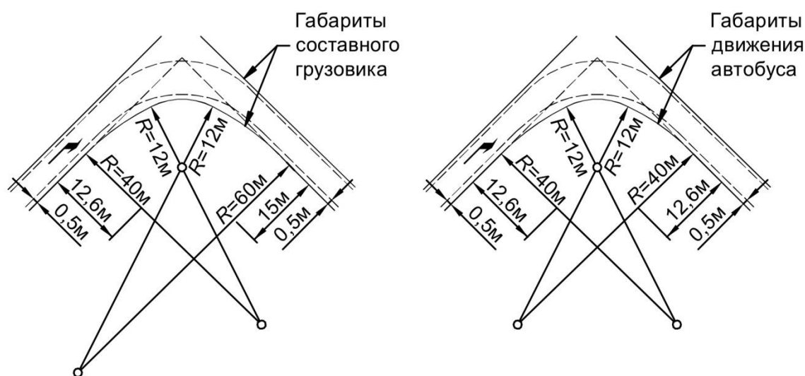
Рисунок Д.2 - Пример построения закругления с серией круговых кривых из трех частей
