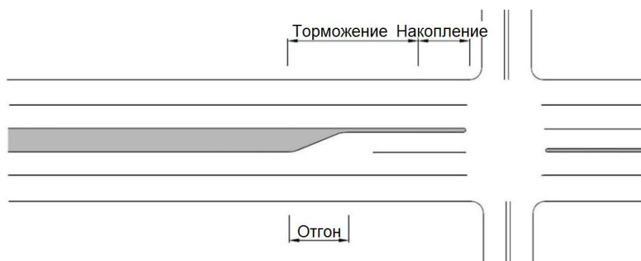
Рисунок 9 – Полоса для поворота налево при наличии центральной разделительной полосы
