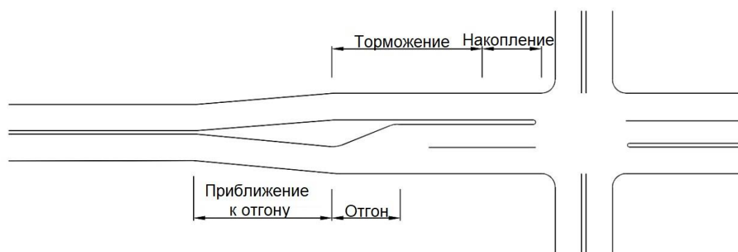
Рисунок 11 – Принципиальная схема отгона полосы для поворота налево на главной дороге
