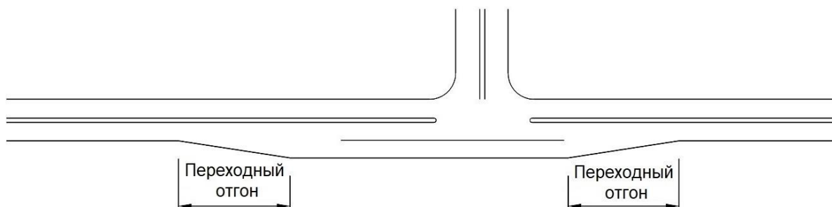
Рисунок 13 – Принципиальная схема построения полосы для поворота налево на главной дороге при низкой интенсивности движения
