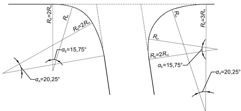
Рисунок Д.3 – Пример построения закругления с серией круговых кривых из трех частей
