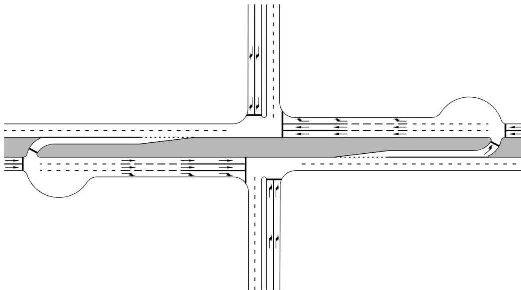
Рисунок 19 – Схема пересечения в одном уровне с отнесенными левыми поворотами с недостаточной для разворота шириной центральной разделительной полосы
