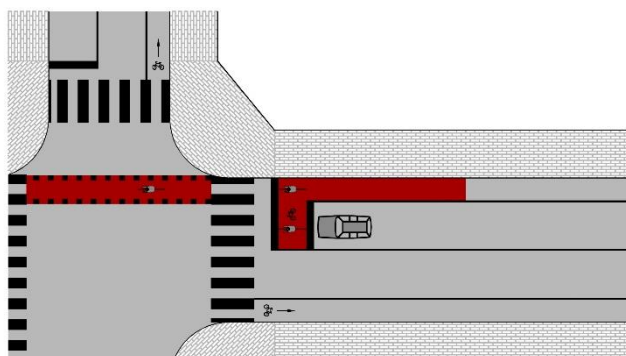
Рисунок 25 – Зона для накопления велосипедистов, ожидающих возможности совершить левый поворот, на двухполосной дороге
