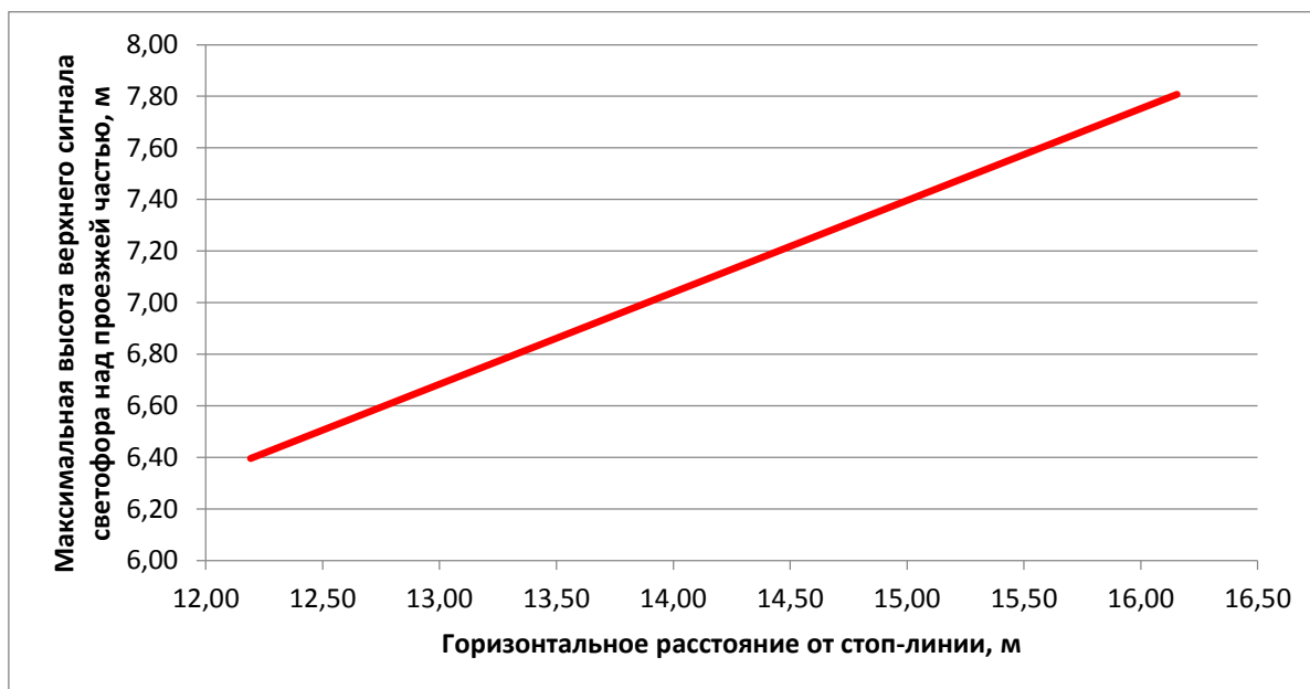
Рисунок В.2 – Максимальная высота установки верхнего сигнала светофора над проезжей частью в зависимости от расстояния до стоп – линии
