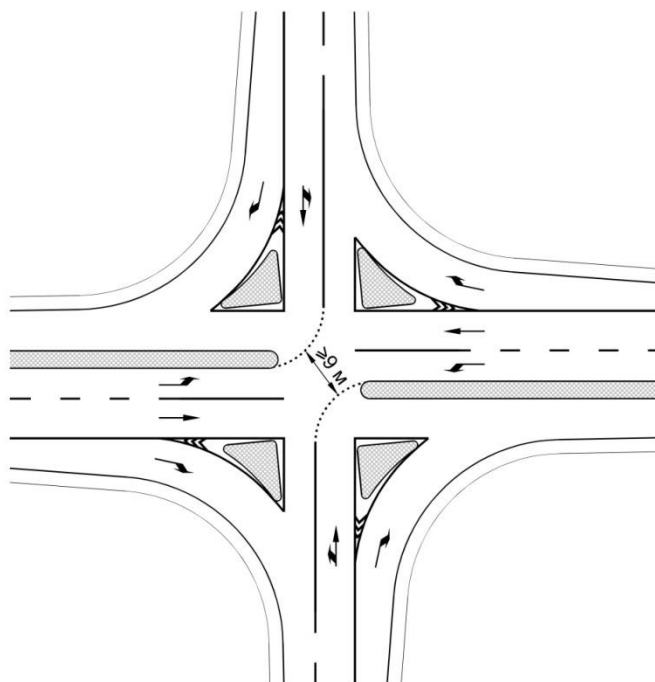
Рисунок 15 – Организация движения при одновременном левом повороте с противоположных направлений
