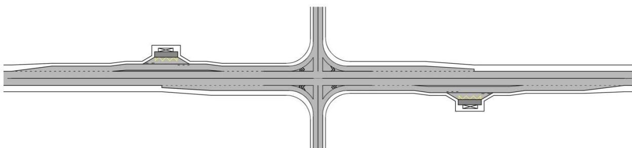
Рисунок 27 - Пример расположения автобусных остановок вблизи пересечения
