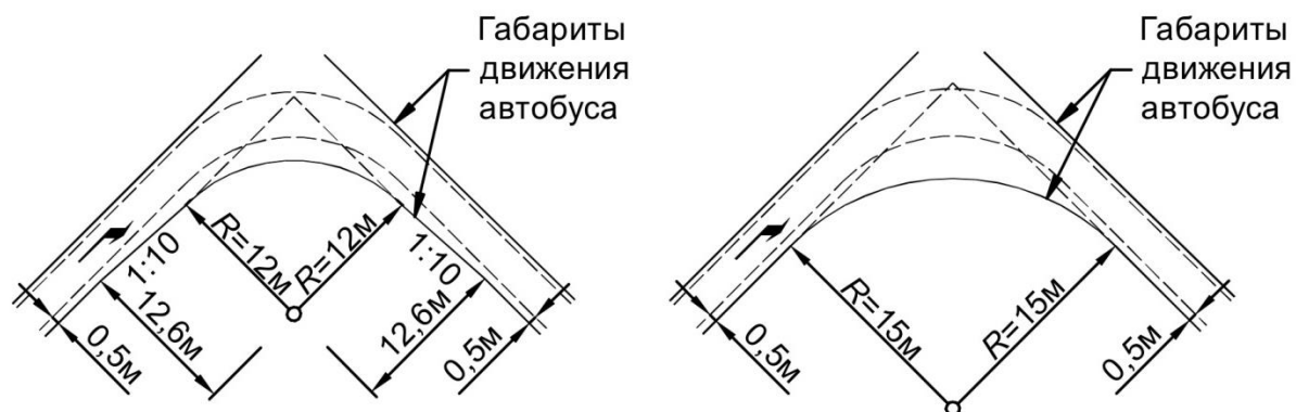
Рисунок Д.1 – Пример построения закругления с отгонами уширения и с единой круговой кривой
