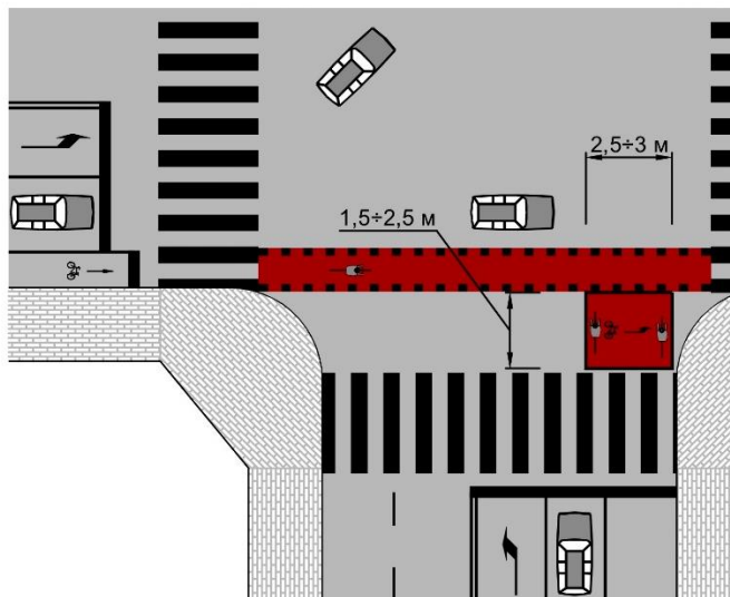
Рисунок 24 – Зона для накопления велосипедистов, ожидающих возможности совершить левый поворот
