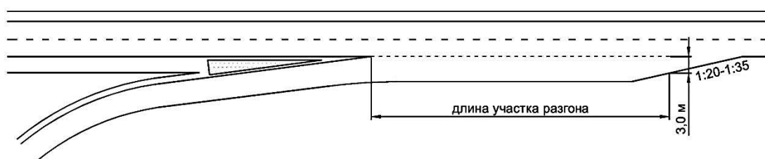
(б) Параллельная полоса разгона
